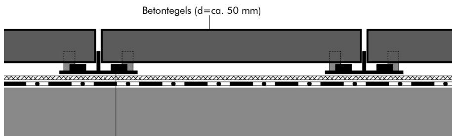
Elastoring - Ringvormige tegeldrager Hoogte ca. 5, 10, 15 or 20 mm
